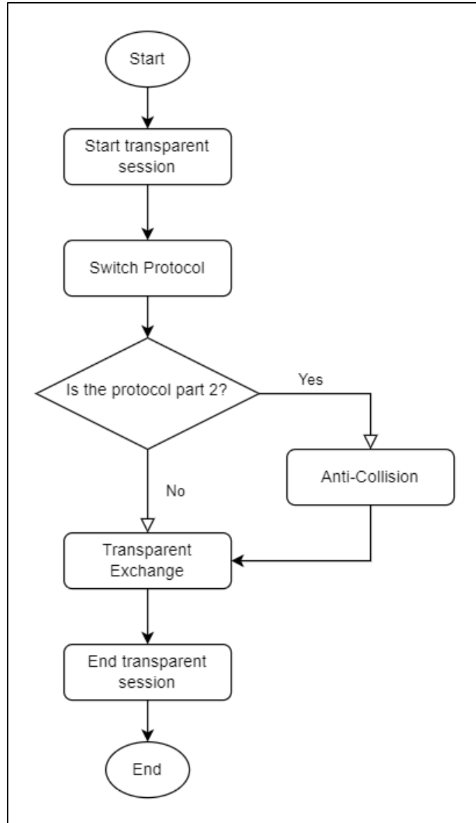
図8 : 透過セッションフローチャート
