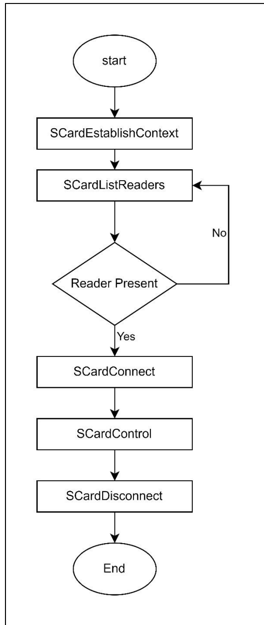
図7 : ACR1555U 直接コマンドの流れ
